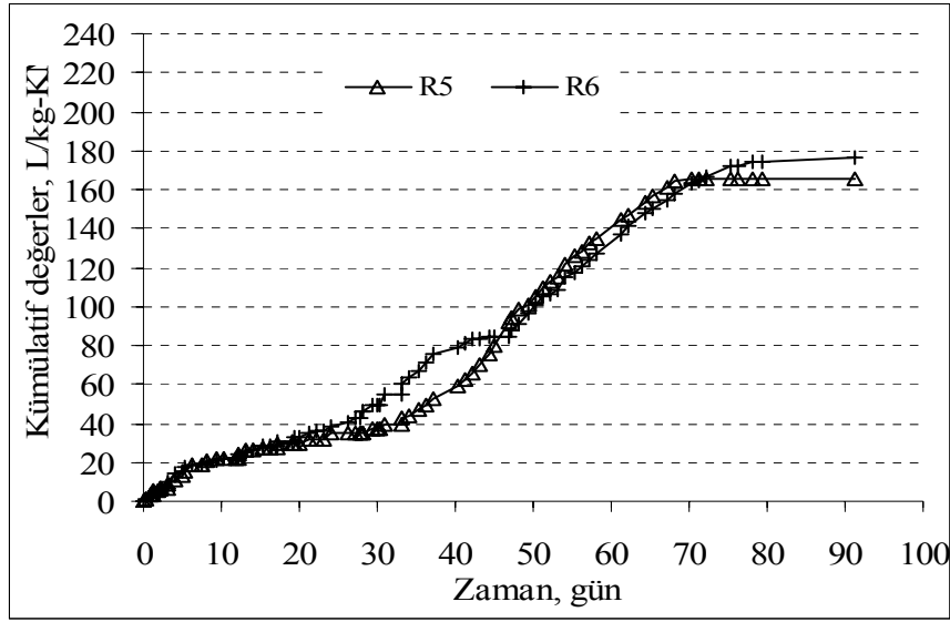
Şekil 4. 5 R5 ve R6 Reaktörlerinde oluşan kümülatif biyogaz değerleri (KM oranı %10, Aşı oranları sırasıyla %0 ve %2,5)
