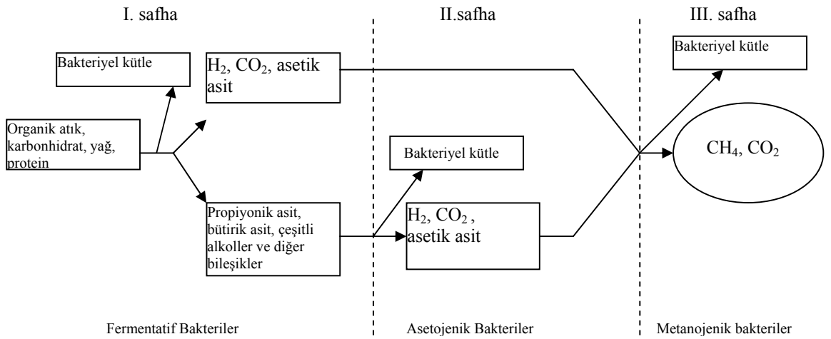
Şekil 2. 2 Anaerobik Çürümenin Safhaları (Kossmann ve Pönitz, 1999'den)
