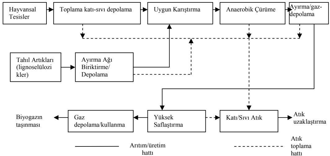
Şekil 2. 1 Tahıl atıklarından gelen lignoselüloziklerle karıştırılan hayvansal atık ve gübreden biyogaz üretim prosesi ( Batzias vd., 2005)
